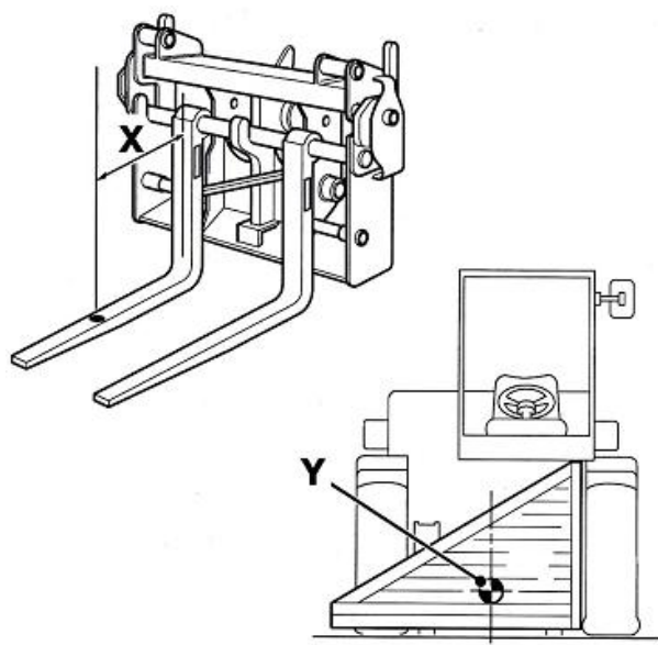
Рис. 2- 26 Центр тяжести нагрузки
