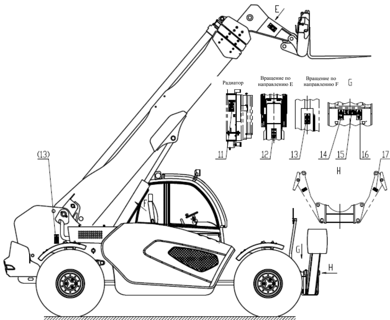
Рис. 1-2 Схема расположения наклеивания предохранительной надписи II
