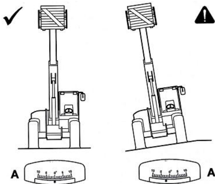
Рис. 2- 47 Подъем на уклоне
