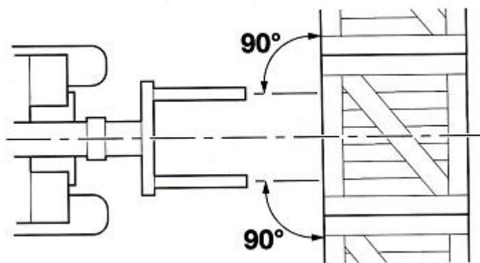
Рис. 2- 34 Схема погрузки
