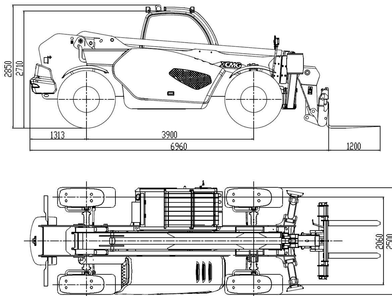
Рис. 4- 3. Диаграмма параметров о габаритном размере погрузчика типа
