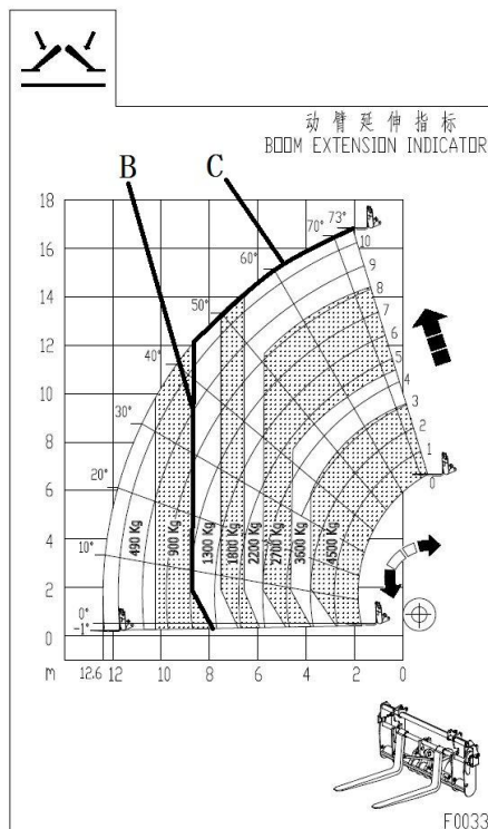
Рис. 2- 27 График нагрузки
