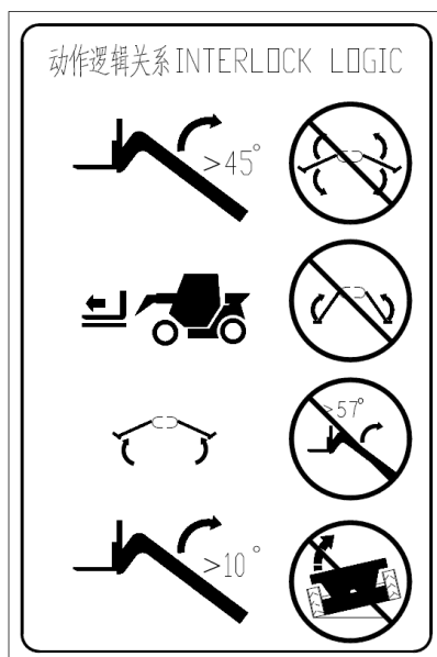
Рис. 2- 24 Логические отношения действия
