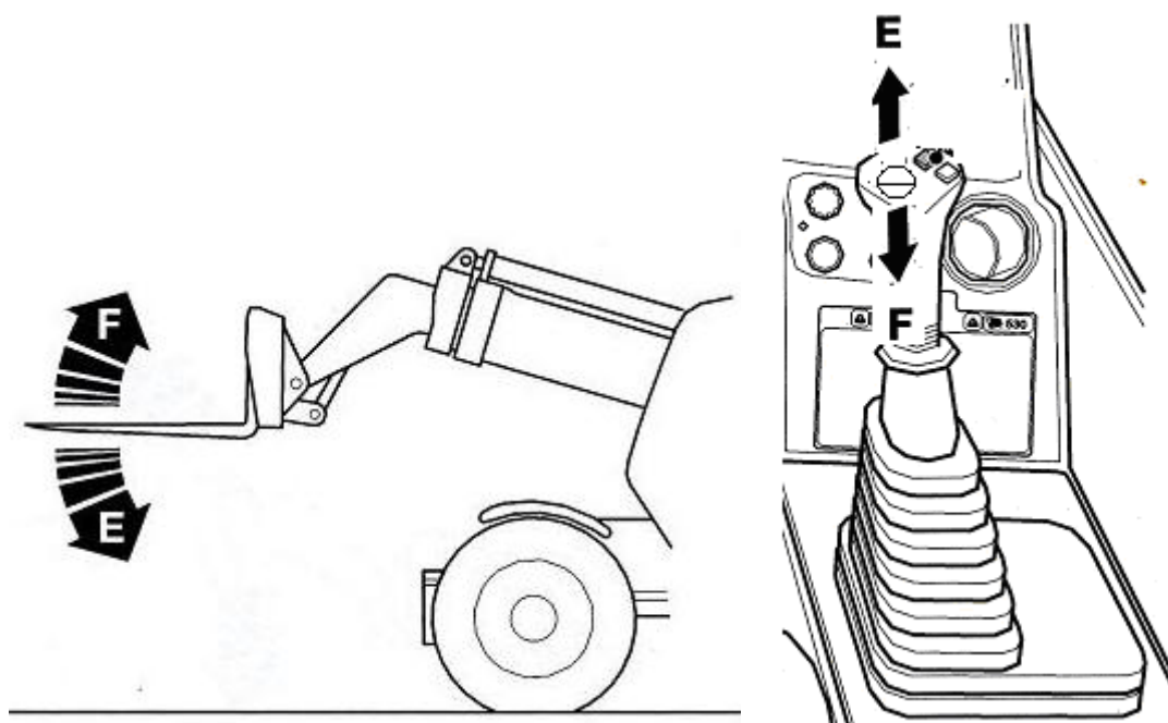
Рис. 2- 18 Втягивание, опрокидывание ковша-лопаты
