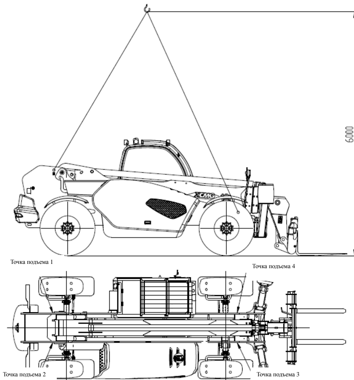
Рис. 2- 51 Подъем вилочного погрузчика
