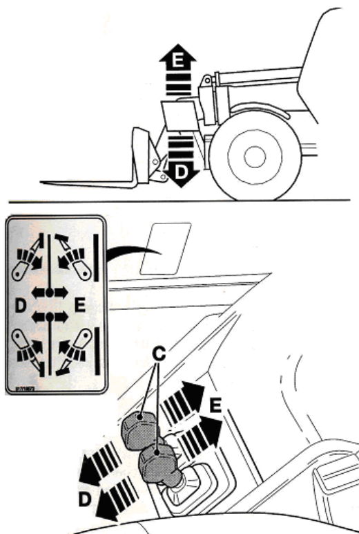
Рис. 2- 23 Управление выносными опорами
