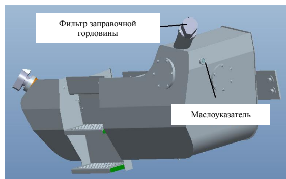
Рис. 3-13 Заправочная горловина гидробака, указатель уровня масла
