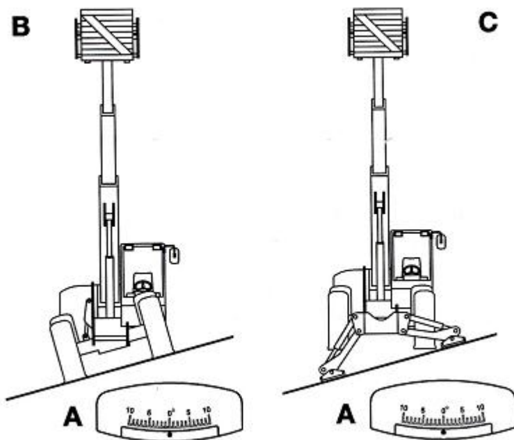
Рис. 2- 46 Подъем на уклоне
