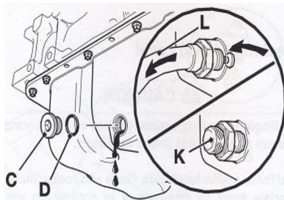
Рис. 3- 19 Спускное отверстие моторного масла
