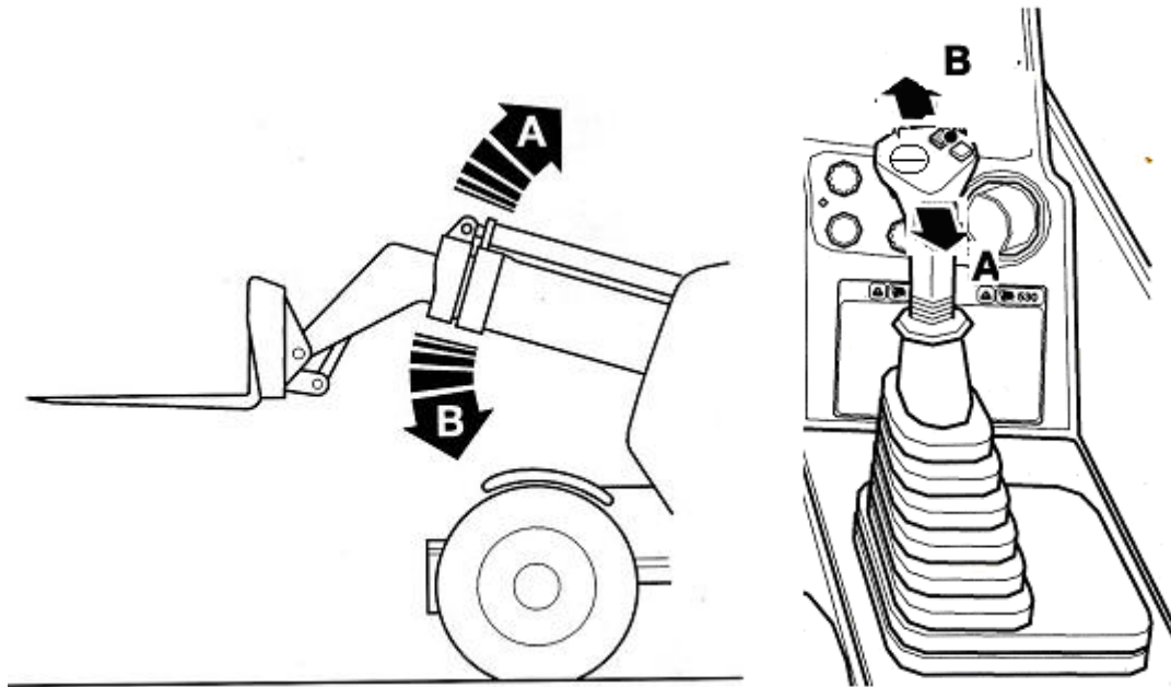
Рис. 2- 16 Подъем/спуск стрелы
