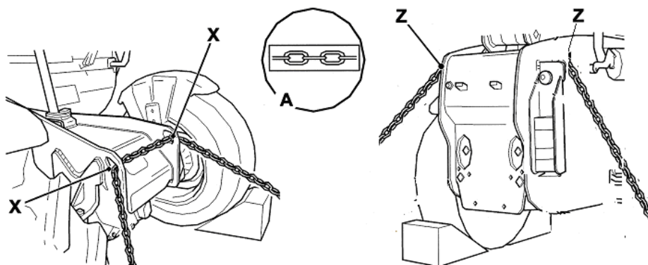
Рис. 2- 50 Транспортировка вилочного погрузчика
