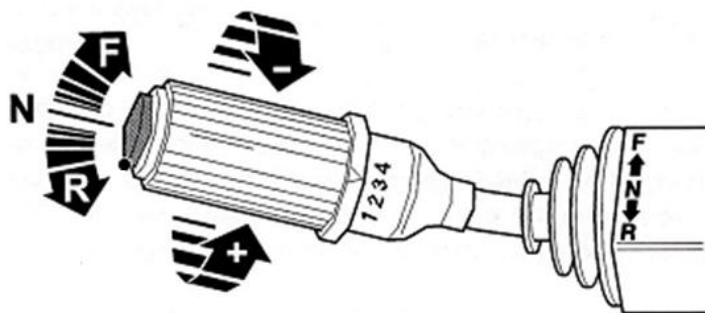
Рис. 2- 9 Схема регулирования рукоятки управления передачами
