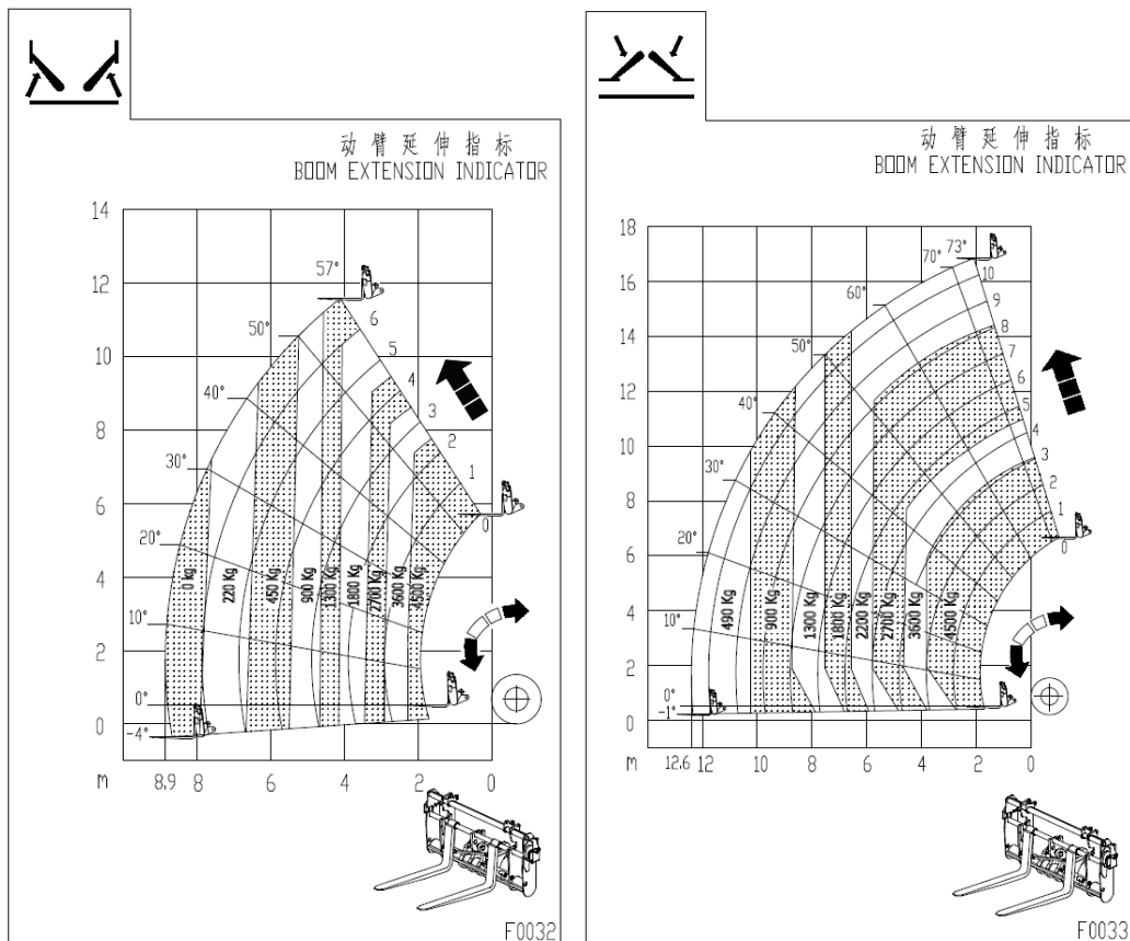
Рис. 2- 25 График нагрузок
