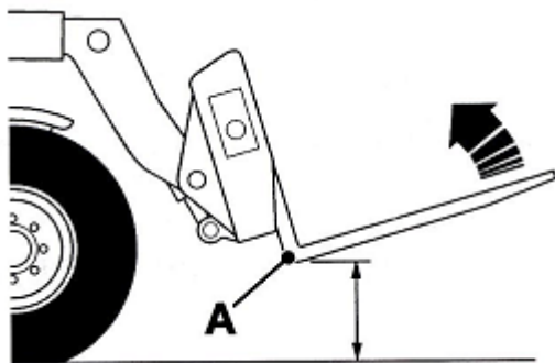
Рис. 2- 29 Втягивание погрузочной вилки
