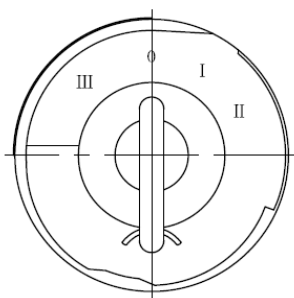
Рис. 2- 12 Пусковой выключатель
